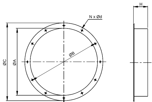
L-Flange
